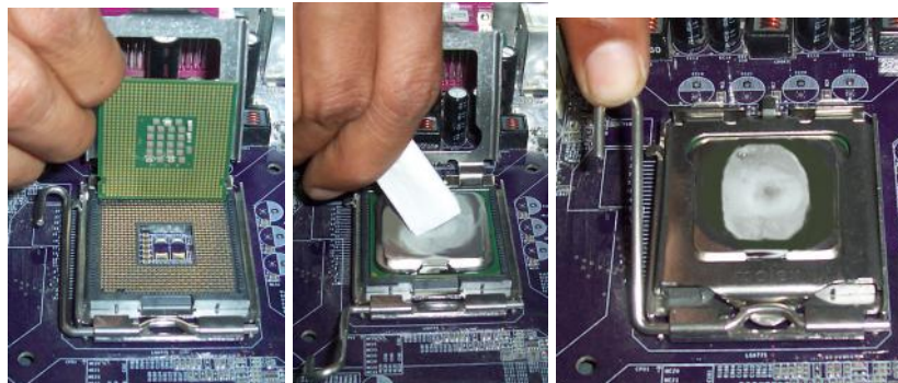
Gambar 3. 6. Pemasangan Prosesor
