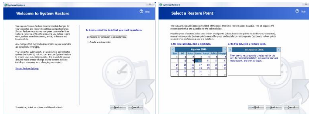
Gambar 7.4. System Restore
