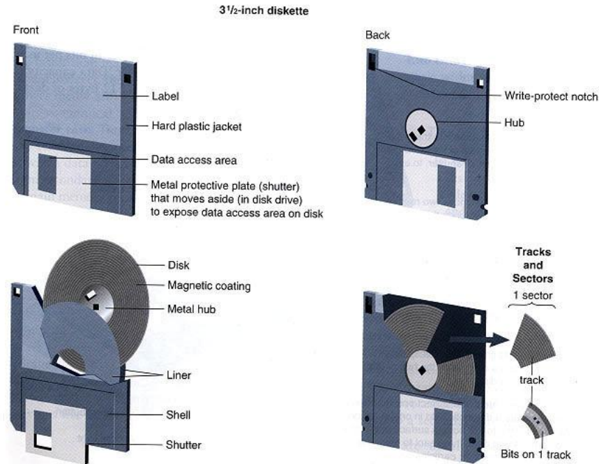
Gambar 2. 25. Floppy disk
